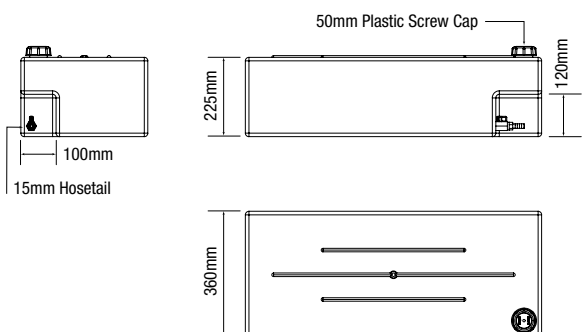
IWT007 - 60L TANK
